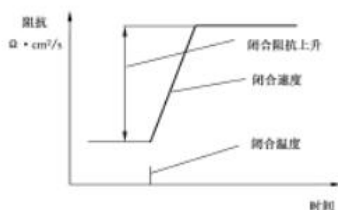
b) 隔膜材料临界状态下闭合电阻上升速度的示意图
