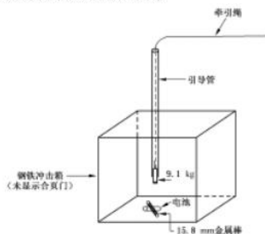
图 E.1 重物冲击试验工装示意图
