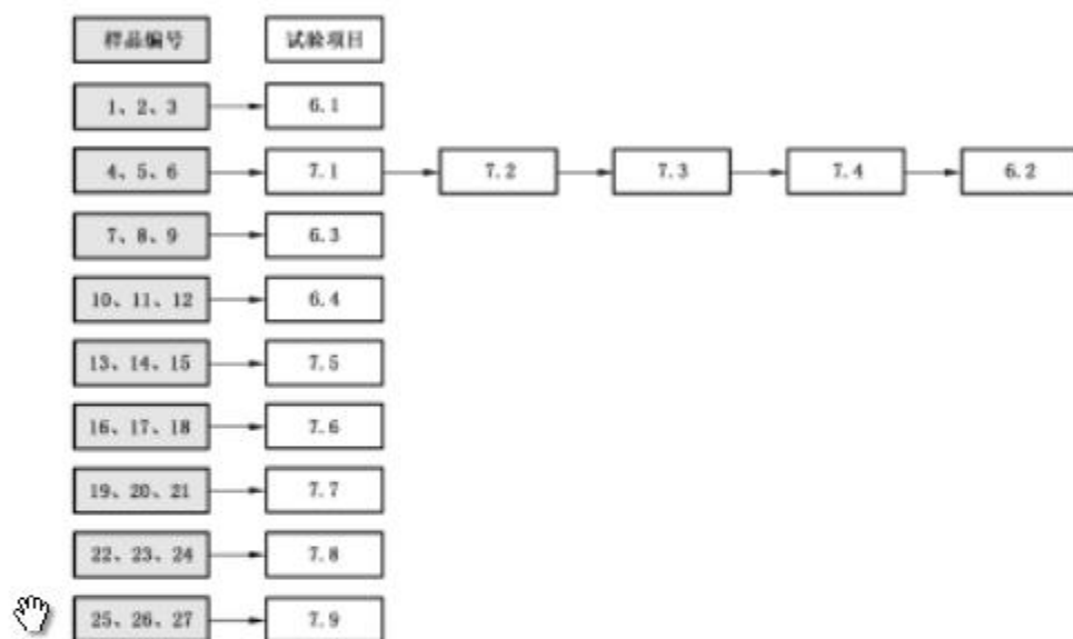
图 C.1 电池安全型式试验顺序
