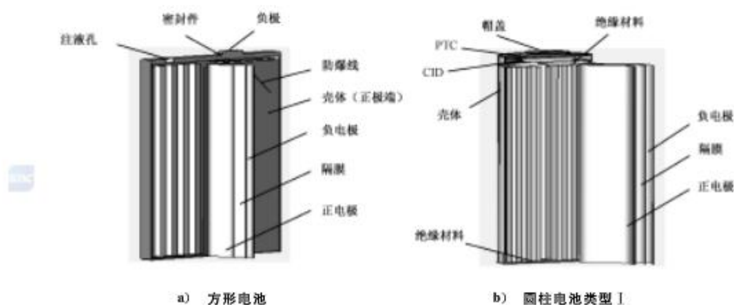
图 B.2 锂离子电池结构实例
