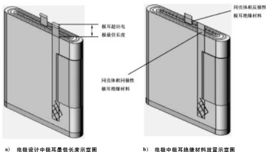
图 B.3 电极中极耳布局
